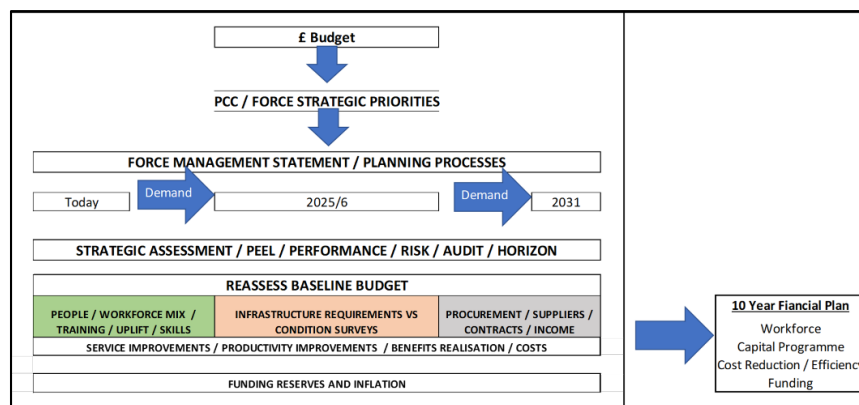
Ffigur 8: Lleoliad Monitro Ariannol a chyswllt â'r Cynllun Ariannol Tymor Canolig
