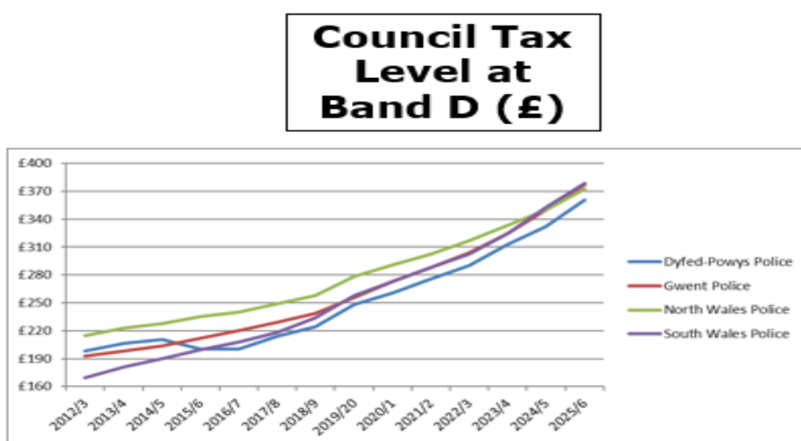
Ffigur 4: Lefelau treth gyngor Cymru
